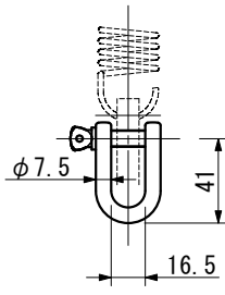
[A] SHACKLE シャックル
